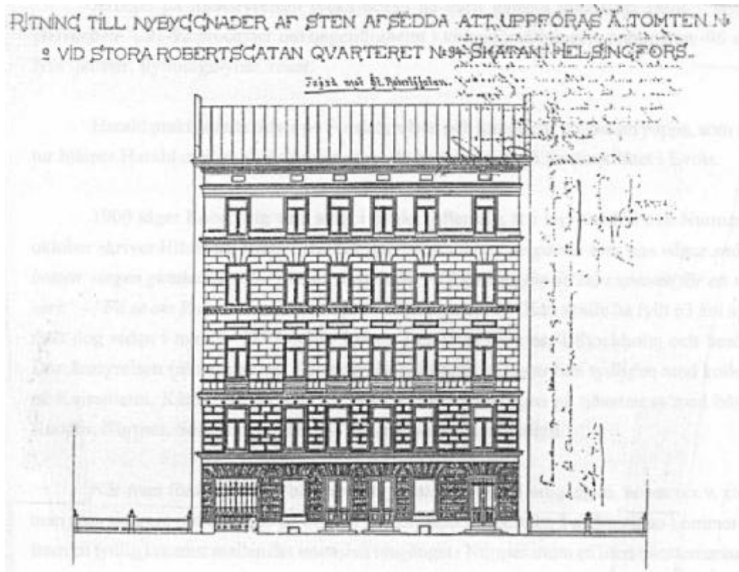
Bild 17. Ritning av fasaden till huset vid Stora Robertsgatan 4. - Stadsarkivet.
